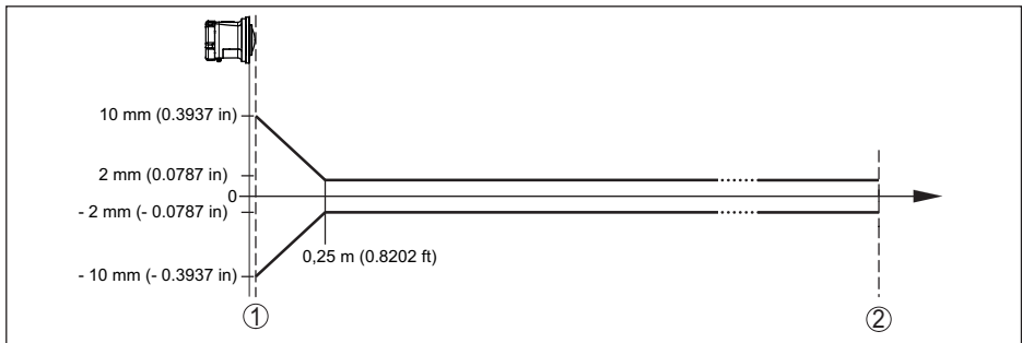
Fig. 21: Error de medición bajo condiciones de referencia
