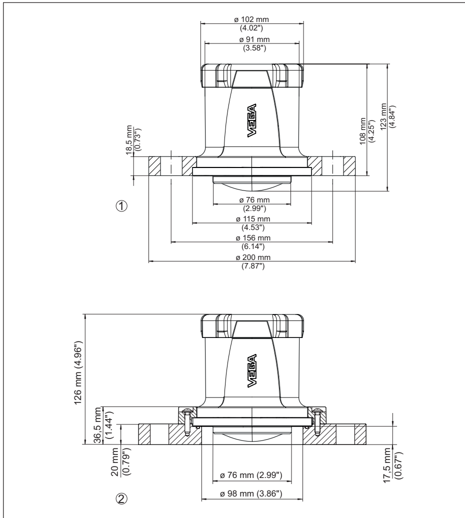
Fig. 22: Medidas VEGAPULS Air 42
