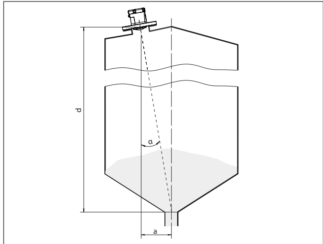
Fig. 12: Propuesta de montaje después de la orientación VEGAPULS Air 42
