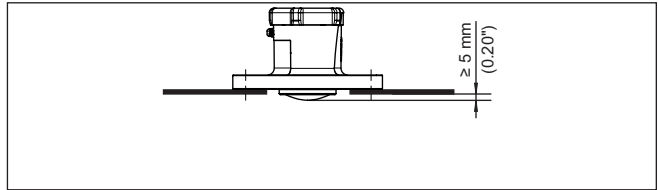
Fig. 8: Montaje recomendado en tubuladura del VEGAPULS Air 42
