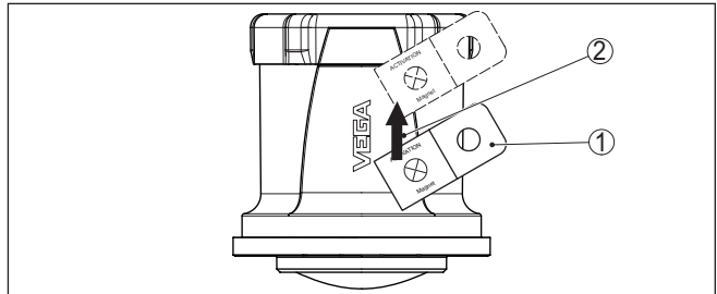
Fig. 14: Activación del sensor mediante imán
