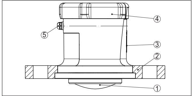
Fig. 1: Componentes del sensor VEGAPULS Air 42 (ejemplo versión mit brida de compresión DN 80)
