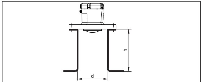
Fig. 9: Montaje de tubuladuras con medidas divergentes
