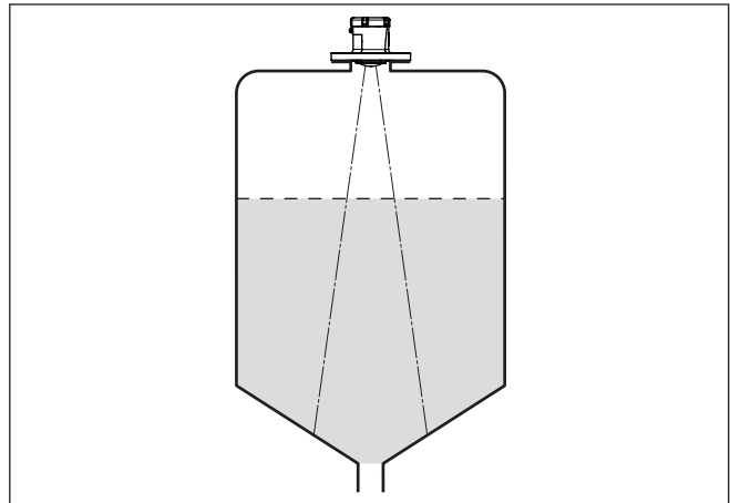
Fig. 6: Montaje del sensor de radar en depósito con fondo cónico
